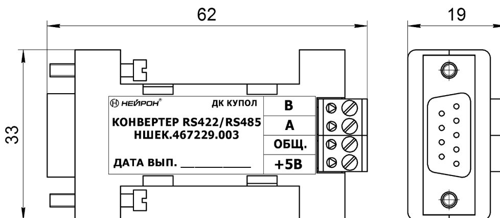
Рис.1 Внешний вид Конвертер RS422/RS485 НШЕК.467229.003
